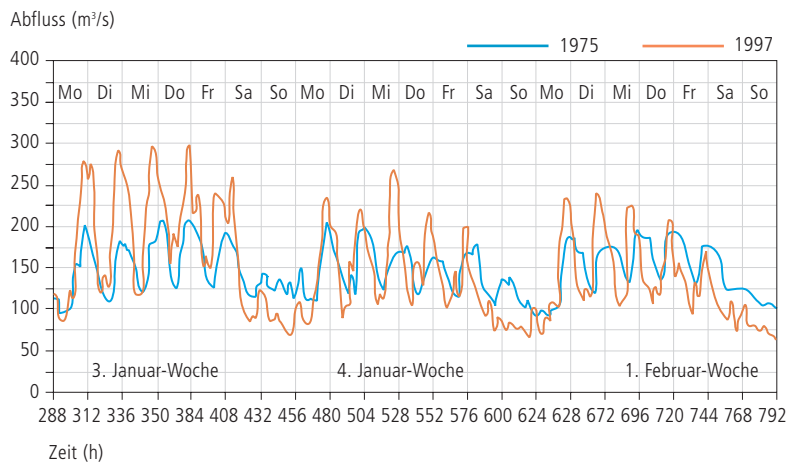
Veränderungen der Schwall-Sunkamplitude bei Diepoldsau zwischen 1975 und 1997 am Beispiel von drei aufeinander folgenden Kalenderwochen im Januar und Februar
