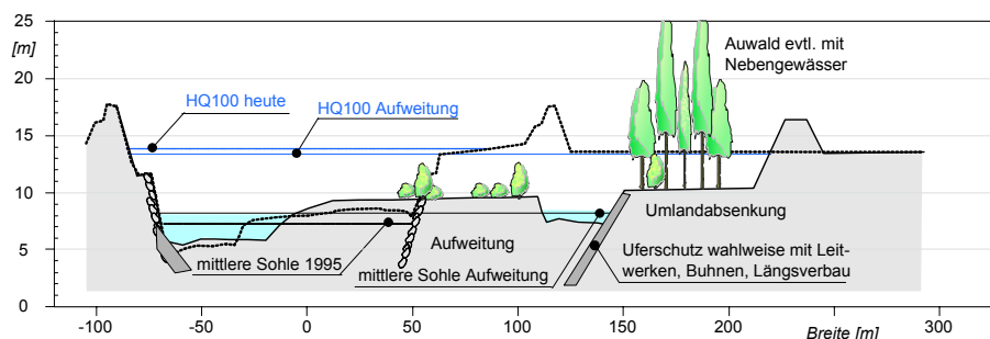
Bild 72: Beispiel einer Umlandabsenkung in Kombination mit einer Flussbettverbreiterung (überhöhte Darstellung)
