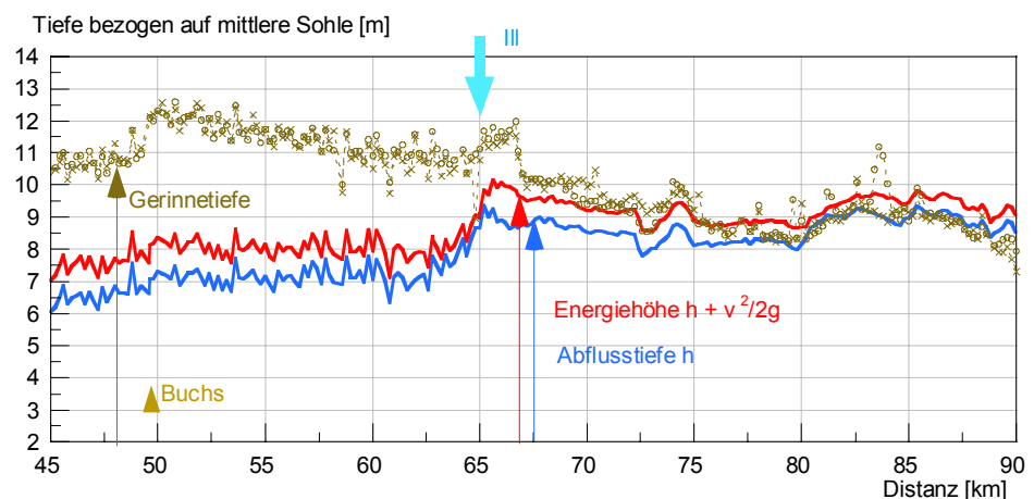
Bild 25: Gerinnetiefe im Vergleich zur Abflusstiefe und Energiehöhe beim HQ_{300} zwischen Buchs und dem Bodensee
