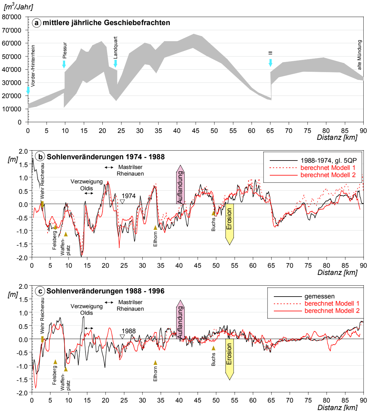
Bild 23: Bandbreite der durchschnittlichen jährlichen Geschiebefrachten, welche im Alpenrhein in der Periode von 1974 bis 1995 transportiert wurden (a), und die gemessenen und berechneten Sohlenveränderungen in der Periode von 1974 bis 1988 (b) und von 1989 bis 1995 (c) für verschiedene Modelle (siehe Detailbericht /5/)
