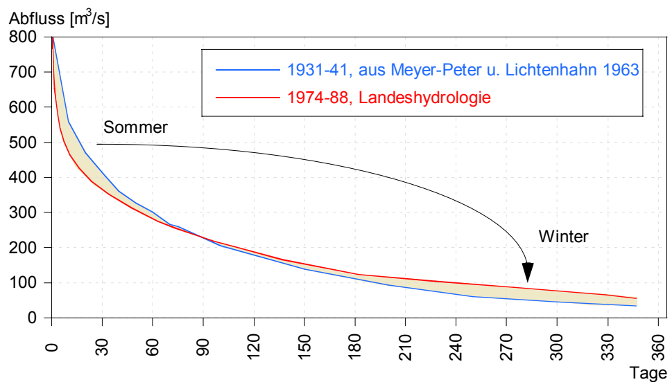
Bild 8: Umlagerung von Sommerabflüssen in den Winter am Beispiel von zwei Dauerkurven bei Bad Ragaz vor und nach dem Kraftwerksbau (Quelle: /1/)
