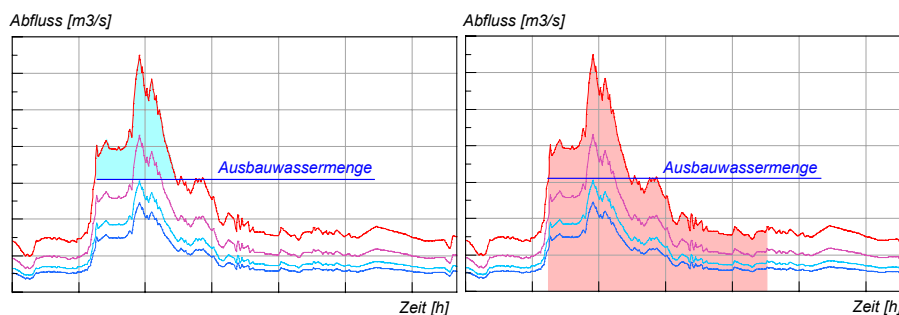
Bild 63: Ohne Massnahmen können im Überlastfall die Dämme brechen und eine grosse Wassermenge fliesst in die Rheintalebene (rote Fläche rechts). Mit einem Überlastfallkonzept können Dammbrüche vermieden und die ausfliessende Wassermenge begrenzt werden (blaue Fläche links).
