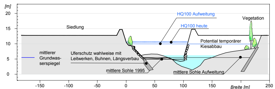
Bild 70: Beispiel einer Verbreiterung des Flussbettes auf 150 m (überhöhte Darstellung)
