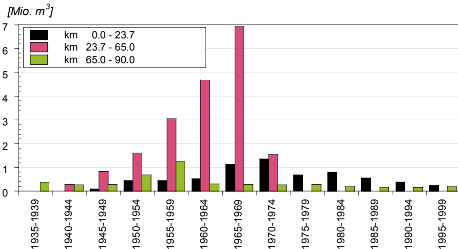
Bild 33: Geschiebeentnahmen im Alpenrhein seit 1936 in verschiedenen Teilstrecken (Erläuterungen siehe Text)
