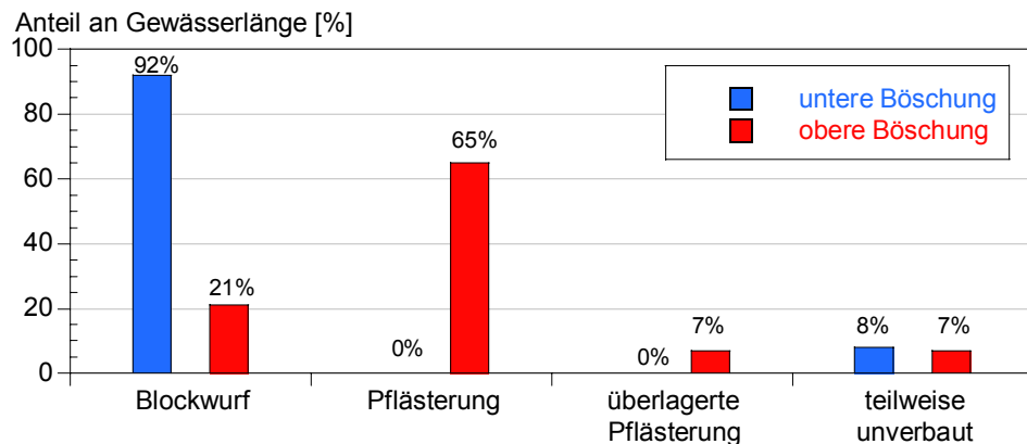
Bild 20: Ufer- und Böschungssicherungen in Prozent der Uferlänge. Linkes und rechtes Ufer sind durchgehend mit grossem, rauem und unverfugtem Blockwurf gesichert. Zumindest teilweise unverbaute Ufer liegen nur mehr in geringem Umfang vor.
