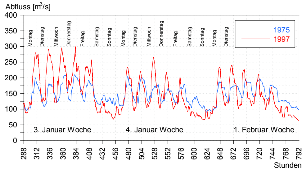
Bild 9: Veränderung der Schwall-Sunkamplitude bei Diepoldsau zwischen 1975 und 1997 am Beispiel von drei aufeinander folgenden Kalenderwochen im Januar und Februar
