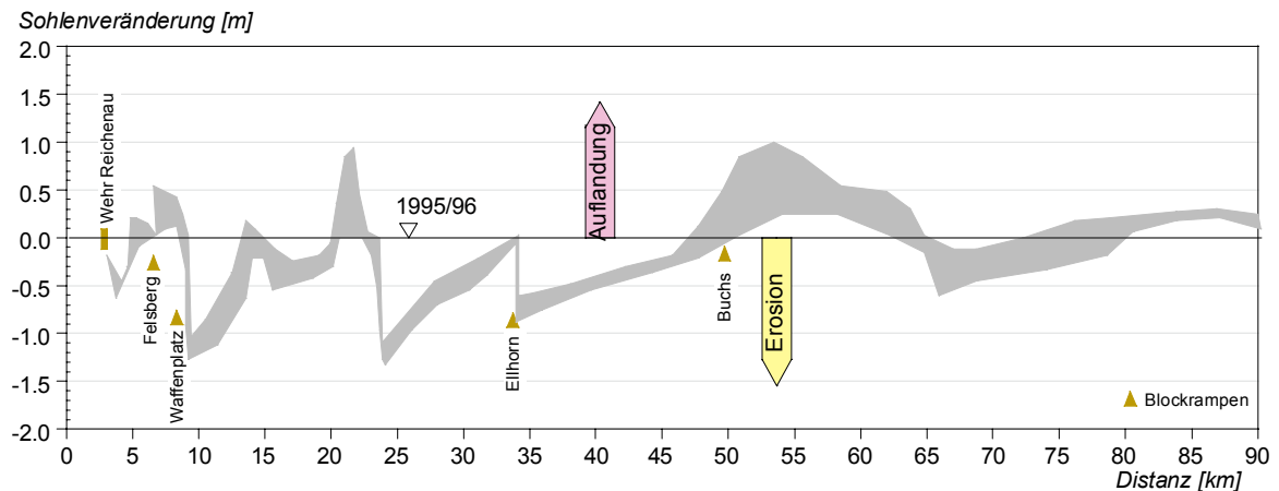
Bild 46: Bandbreite der wahrscheinlichen Sohlenveränderungen in den nächsten 25 Jahren für Bedingungen wie in der Periode von 1974 bis 1995 (gleitendes Mittel über 5 Querprofile)
