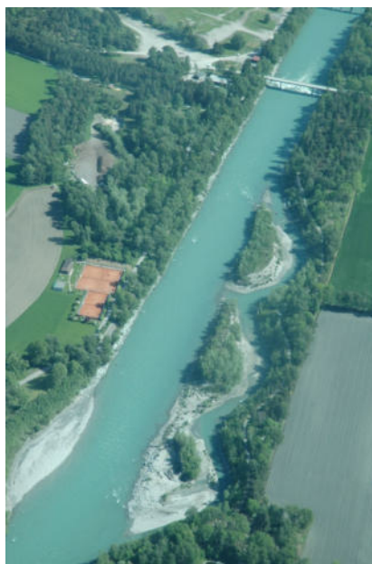
Bild 61: Aufweitung bei Chur/Felsberg, welche 1997 realisiert wurde.
