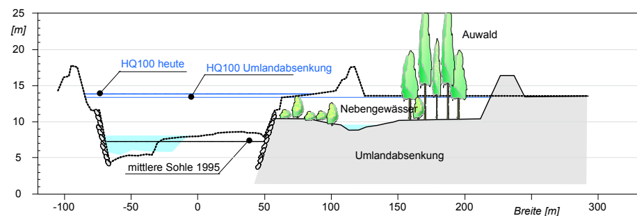
Bild 71: Beispiel einer Umlandabsenkung (überhöhte Darstellung)
