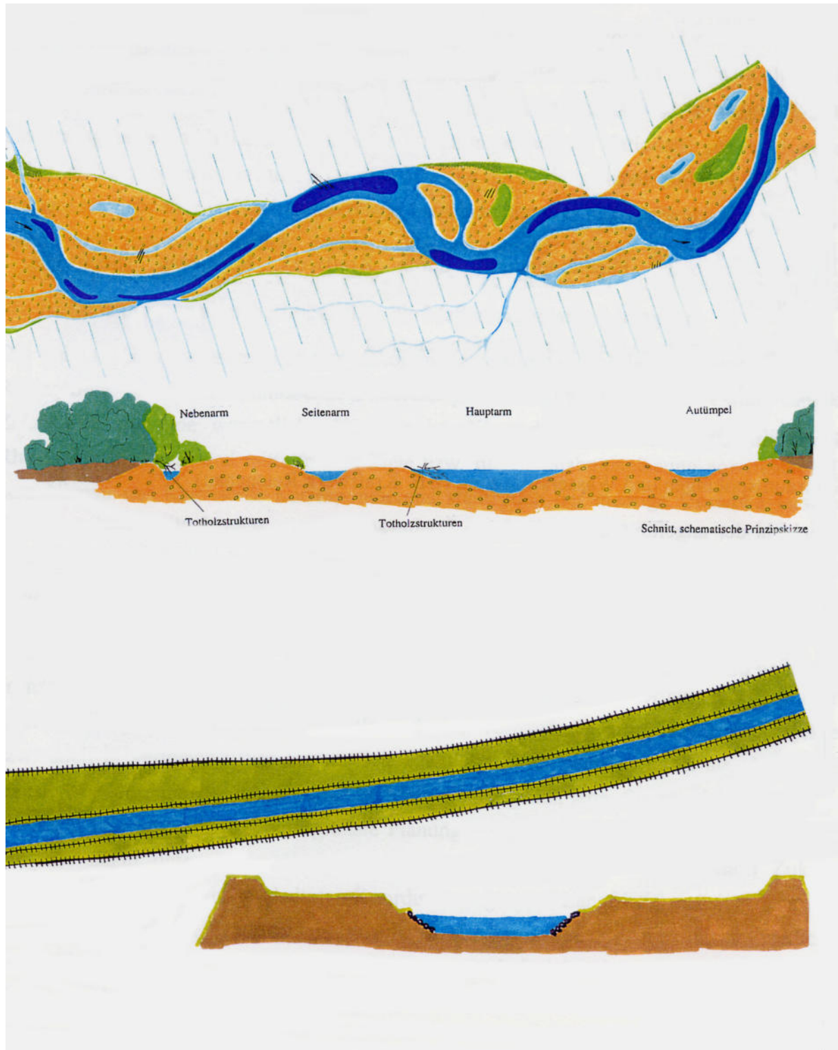
Bild 49: Vergleich Referenzzustand des gewunden-verzweigten Flusstyps zur derzeitigen Situation in der Internationalen Strecke (aus: Gewässer- & fischökologisches Konzept Alpenrhein)
