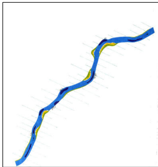
Bild 38: gestreckter Flusslauf
