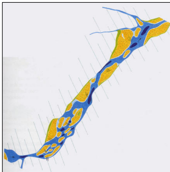
Bild 39: verzweigter Flusslauf
