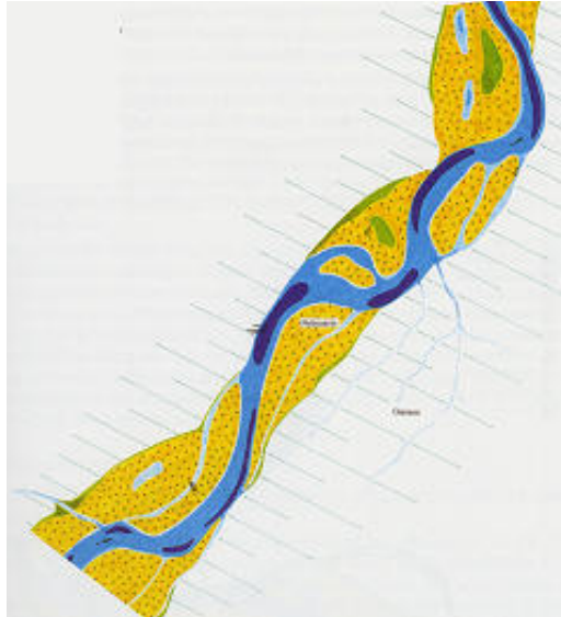
Bild 40: gewunden-verzweigter Flusslauf
