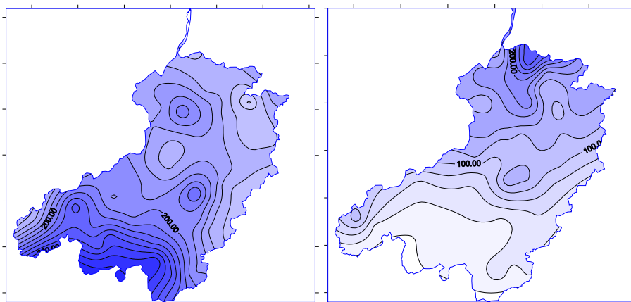
Bild 10: Beispiele von süd- (1987) und nordzentrierten (1910) Niederschlagsfeldern mit grossen Hochwasserabflüssen im Alpenrhein (Quelle: /3/)
