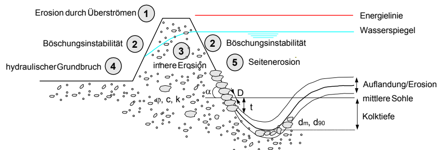
Bild 24: mögliche Versagensprozesse
