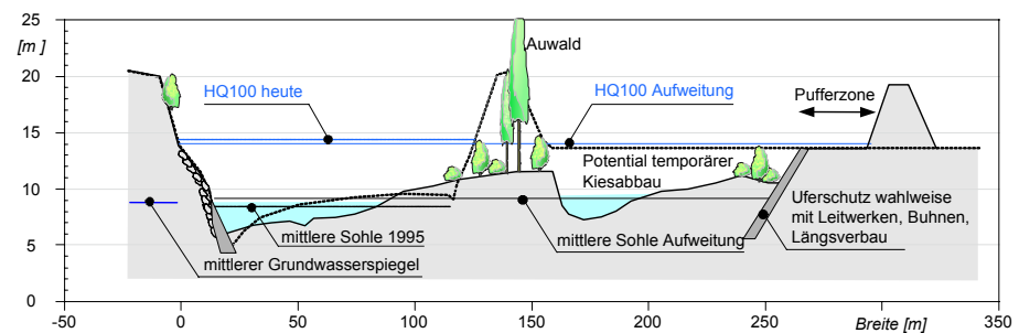
Bild 69: Beispiel einer Verbreiterung des Flussbettes auf 200 m und mehr (oberhalb internationaler Rheinstrecke)
