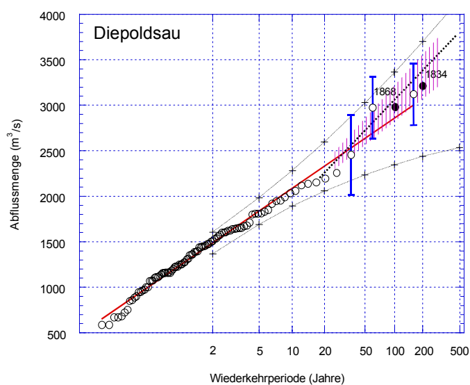
Bild 12: Abflussstatistik der Jahresmaxima in der internationalen Rheinstrecke und die 4 grössten Ereignisse zwischen 1800 und 2000 (Quelle: /3/)
