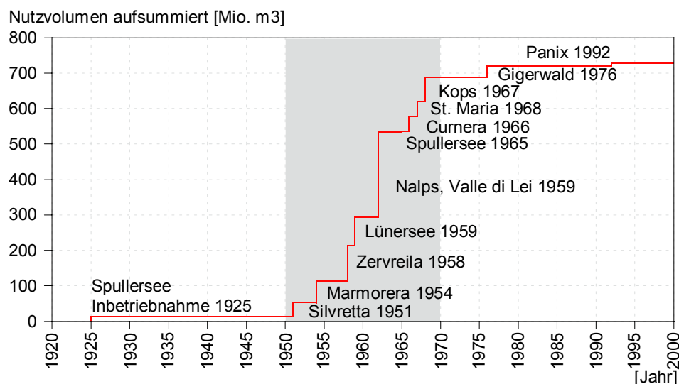
Bild 3: Zunahme des Nutzvolumens der für die Hochwasserretention im Alpenrhein relevanten Speicher (fett markierte Speicher in Bild 2)
