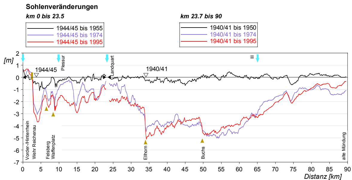
Bild 17: Sohlenveränderungen im Alpenrhein zwischen 1941 und 1995
