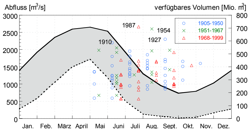
Bild 4: Bandbreite des für die Hochwasserretention im Alpenrhein verfügbaren Volumens der relevanten Speicher (fett markierte Speicher in Bild 2) im Jahresverlauf der Jahresabflussspitzen vor (blau), während (grün) und nach (rot) dem Speicherboom bei Diepoldsau (internationale Rhein-strecke)
