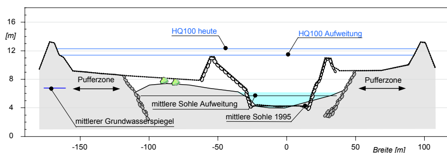
Bild 73: Beispiel einer Aufweitung in der internationalen Rheinstrecke mit beidseitigen Pufferzonen (überhöhte Darstellung)
