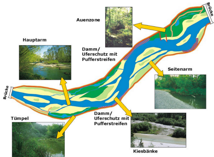
Bild 68: Mögliche Morphologie in einer Aufweitung oberhalb der Illmündung mit Flussbettbreiten von teilweise deutlich über 200 m
