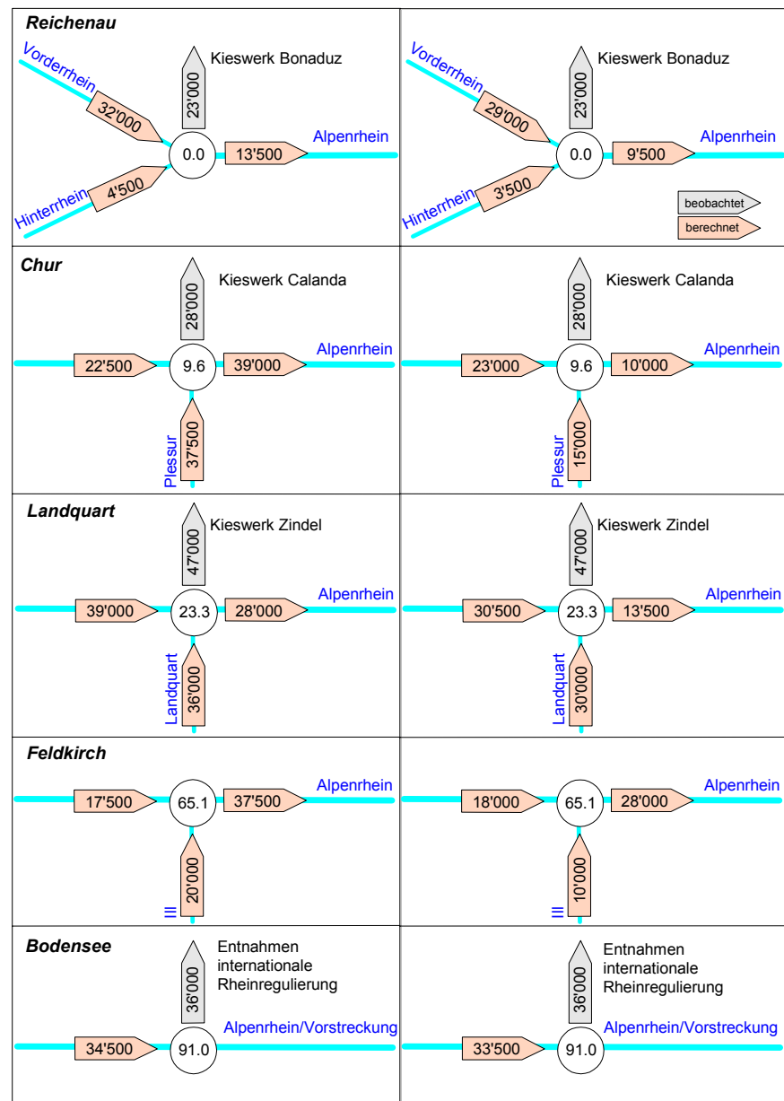
Bild 22: Geschiebebilanzen bei den Mündungen der Zuflüsse und beim Bodensee in m 3 pro Jahr für die Periode von 1974 bis 1995 für das Modell 1 (links) und das Modell 2 (rechts)
