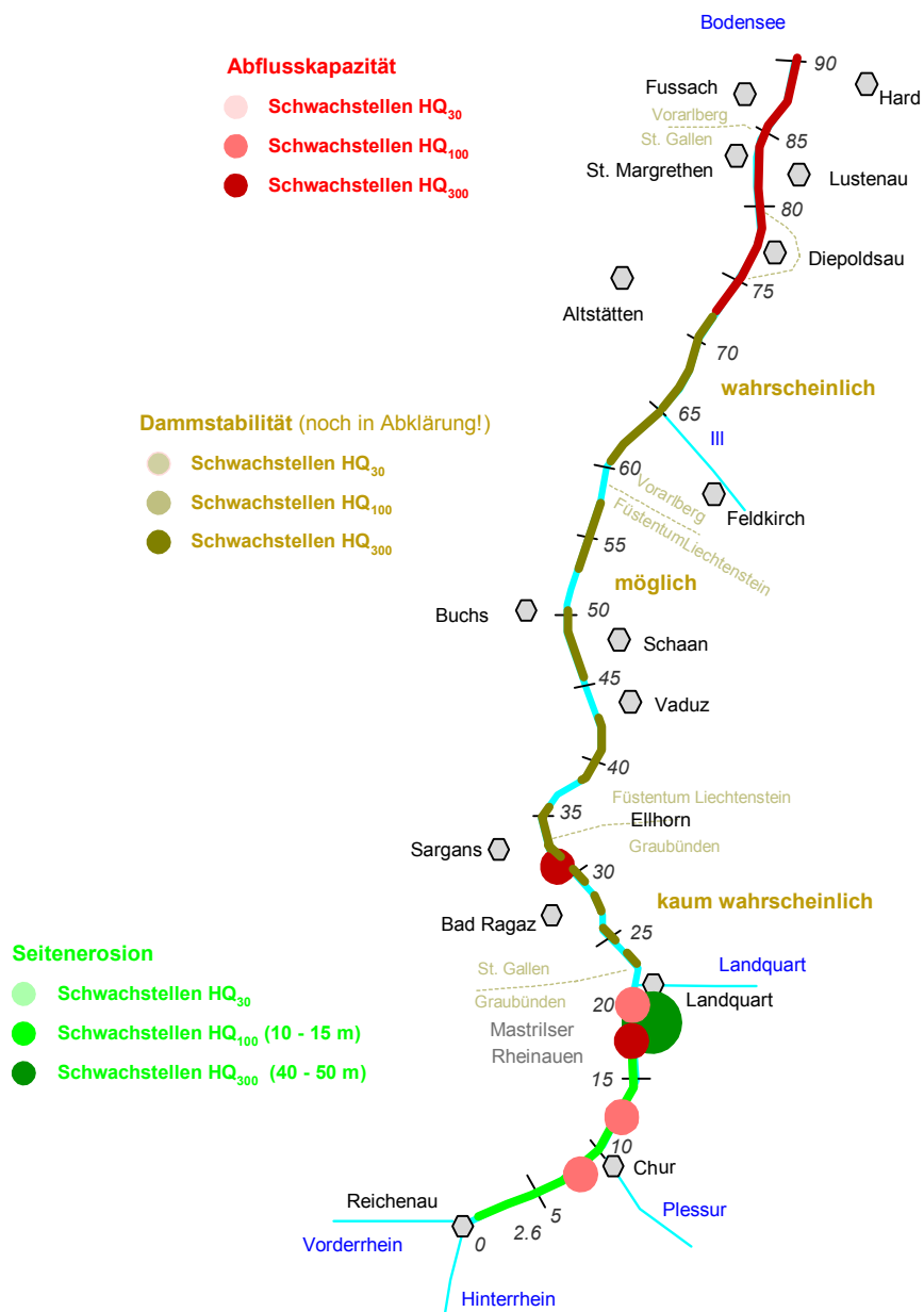
Bild 47: Schwachstellen am Alpenrhein bei Hochwasserereignissen mit unterschiedlichen Jährlichkeiten
