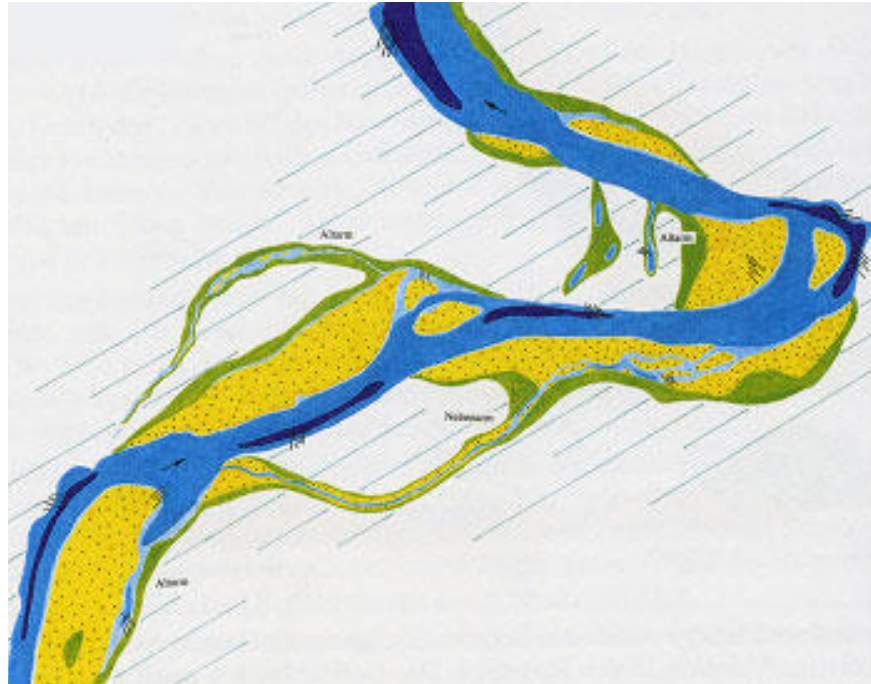
Bild 41: gewundener Flusslauf
