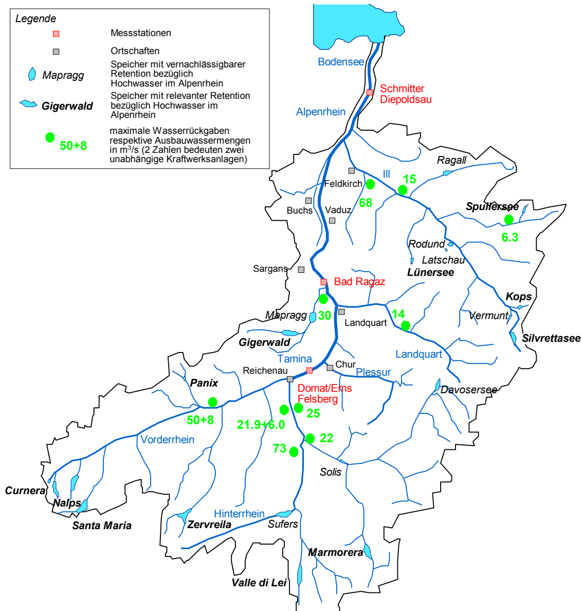
Bild 2: Übersicht über das Einzugsgebiet des Alpenrheins.
