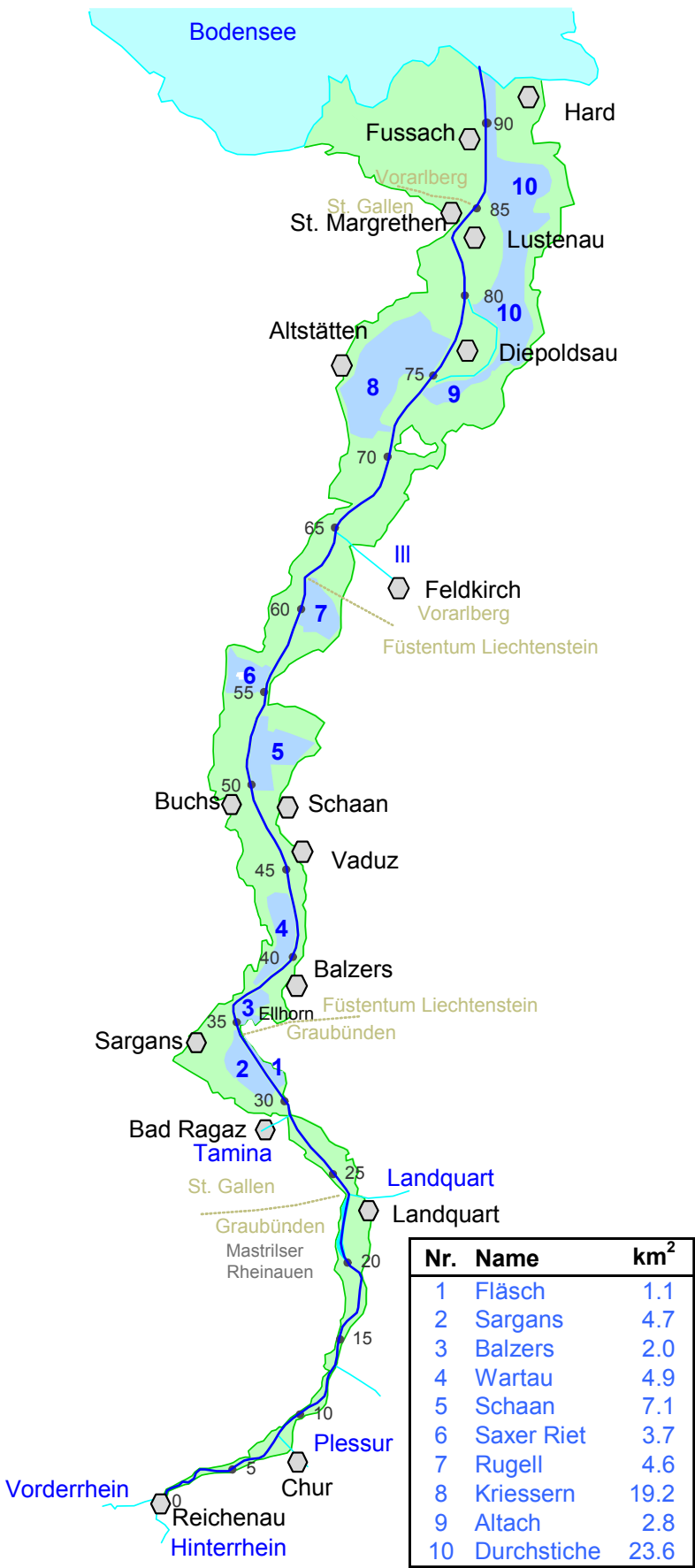
Bild 65: Lage der möglichen Notentlastungsräume und ihre ungefähre Ausdehnung
