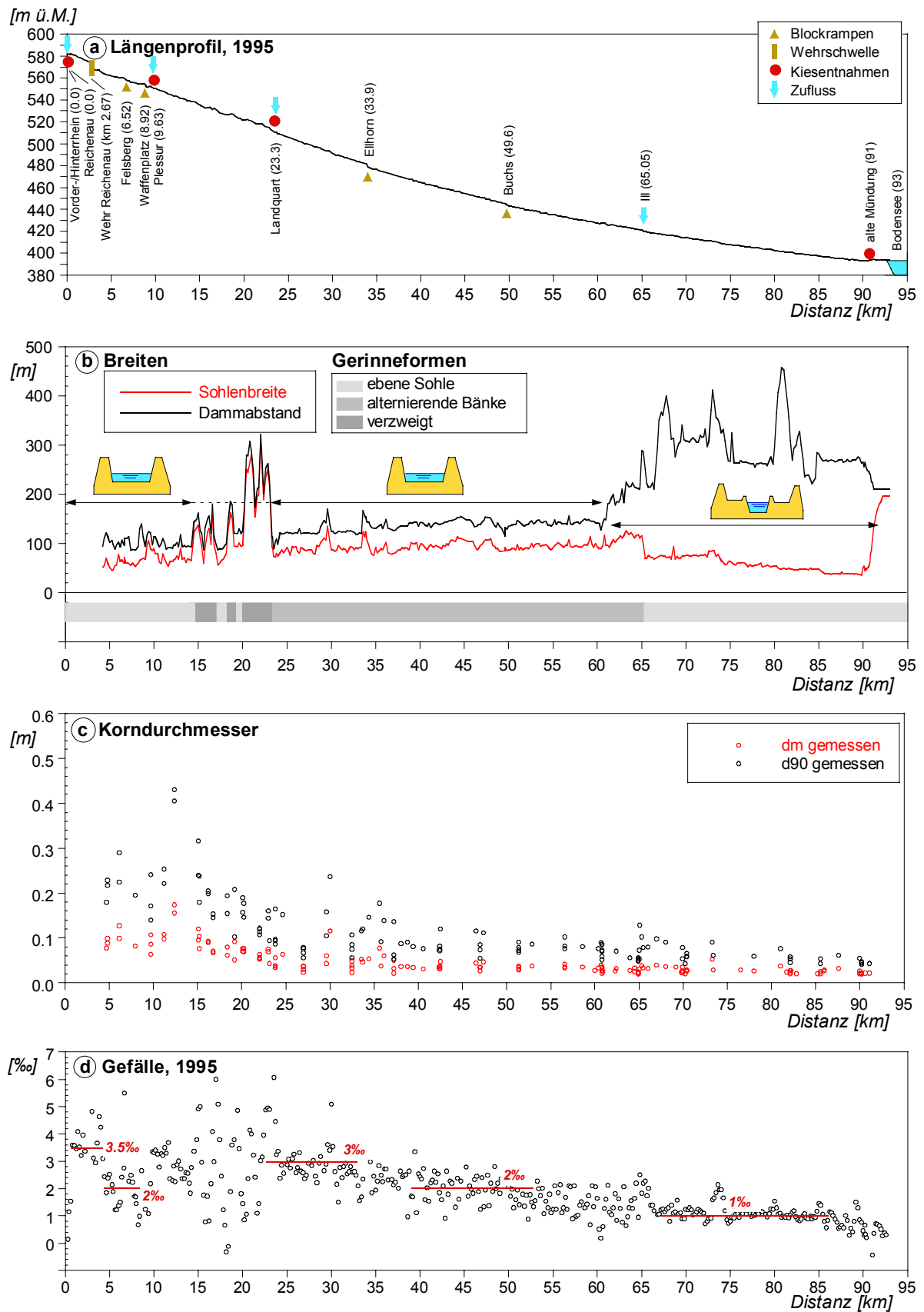
Bild 14: Längenprofil, Flussbettbreite und Abstand der Dämme, charakteristische Korndurchmesser sowie Gefällsverhältnisse des Alpenrheins
